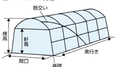
図1 ハウスの構造
