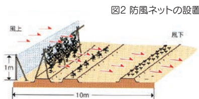
図2 防風ネットの設置
